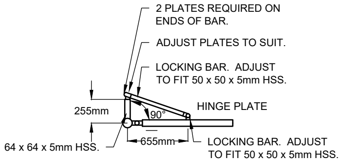
DETAIL A-A
